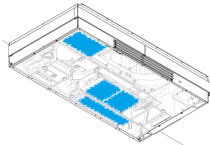
Abbildung 22: Platzierung des Kondensatsystems innerhalb des DUPLEX Vent X
