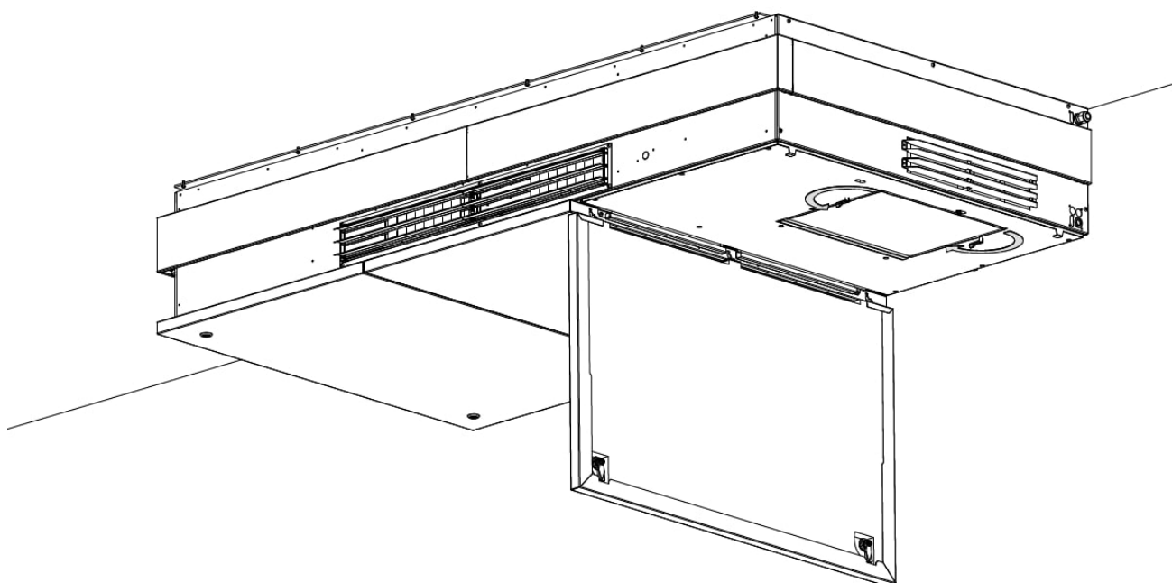
Abbildung 18: Schließen der Filterklappe
