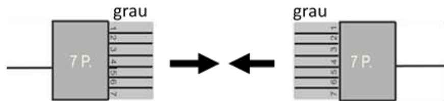
Geräte mit Steuerung RD5 und RD6
