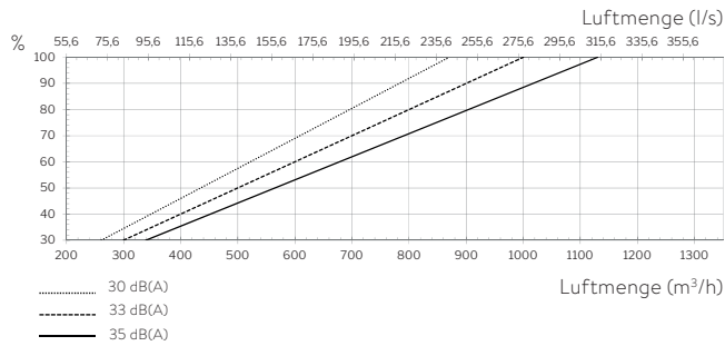
V - L/R KAPAZITÄT mit ePM 10 50% / ePM 10 50% Filter 1
