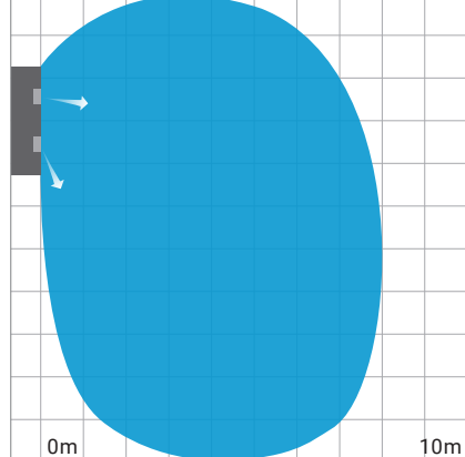
Bei maximaler Luftmenge mit separaten Luftströmen
