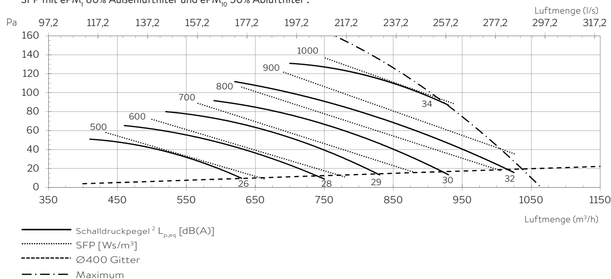
SFP mit ePM 1 80% Außenluftfilter und ePM 10 50% Abluftfilter 3:
