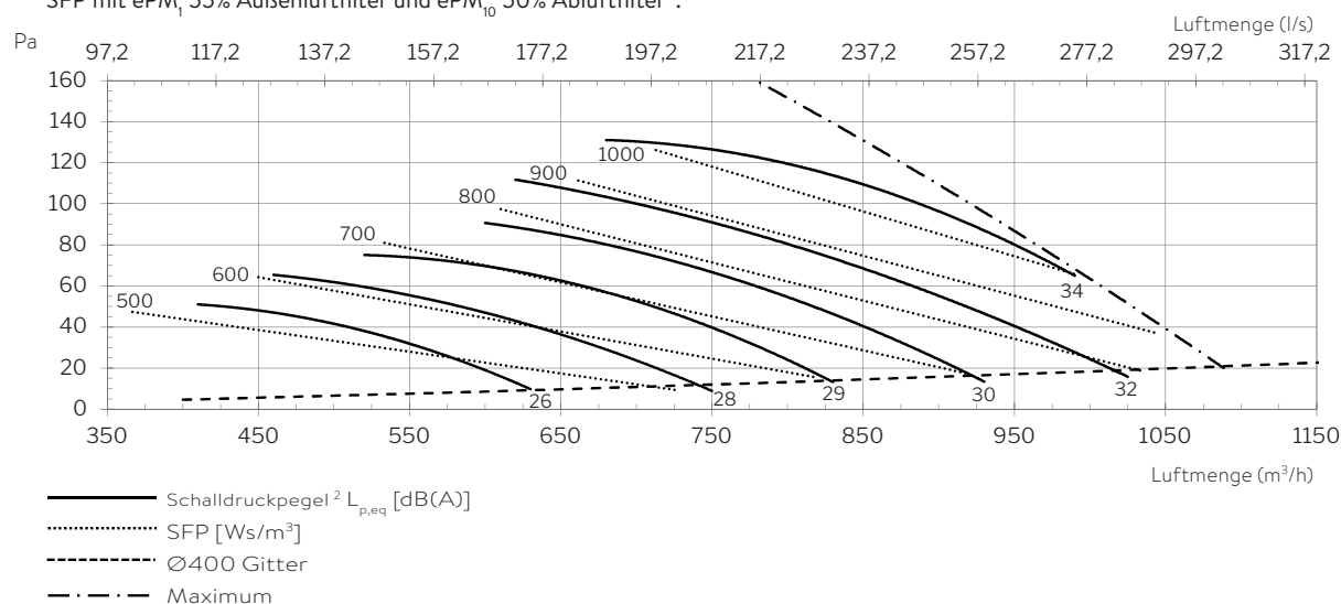
SFP mit ePM 1 55% Außenluftfilter und ePM 10 50% Abluftfilter 2:
