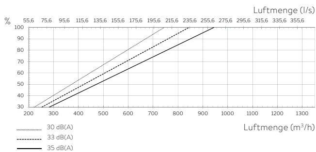
H - L/R KAPAZITÄT mit ePM 1 80% / ePM 10 50% Filter 1
