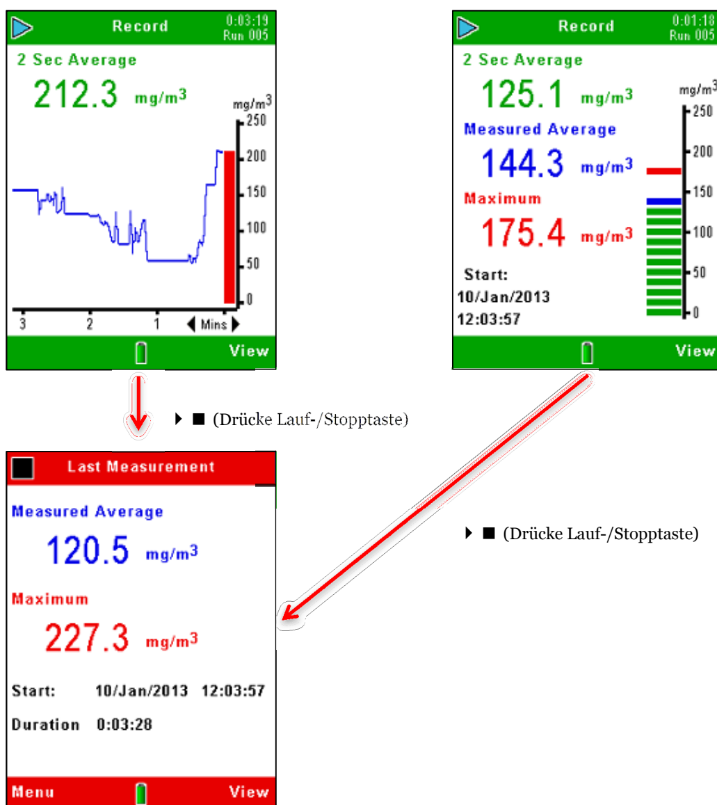
Abbildung 20 Speichern stoppen
