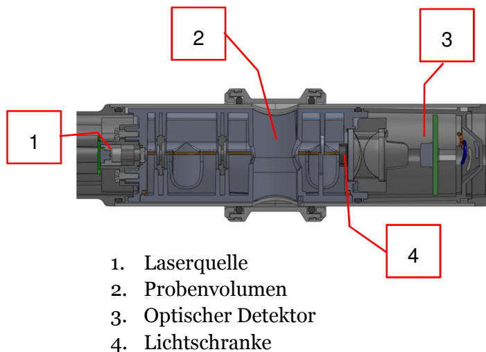
Abbildung 2 Probenahmesonde
