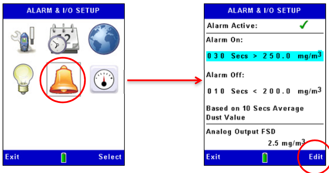
Abbildung 11 Alarmeinrichtung
