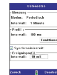
Stellen Sie 2 Pegel der Zeitbilanzspeicherung ein
