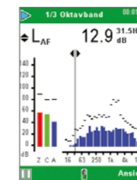
Frequenzanalyse und Einzelmessbereich in Echtzeit
