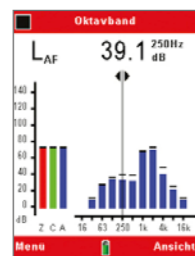
Oktavbandmessungen für die Wahl von PPE
